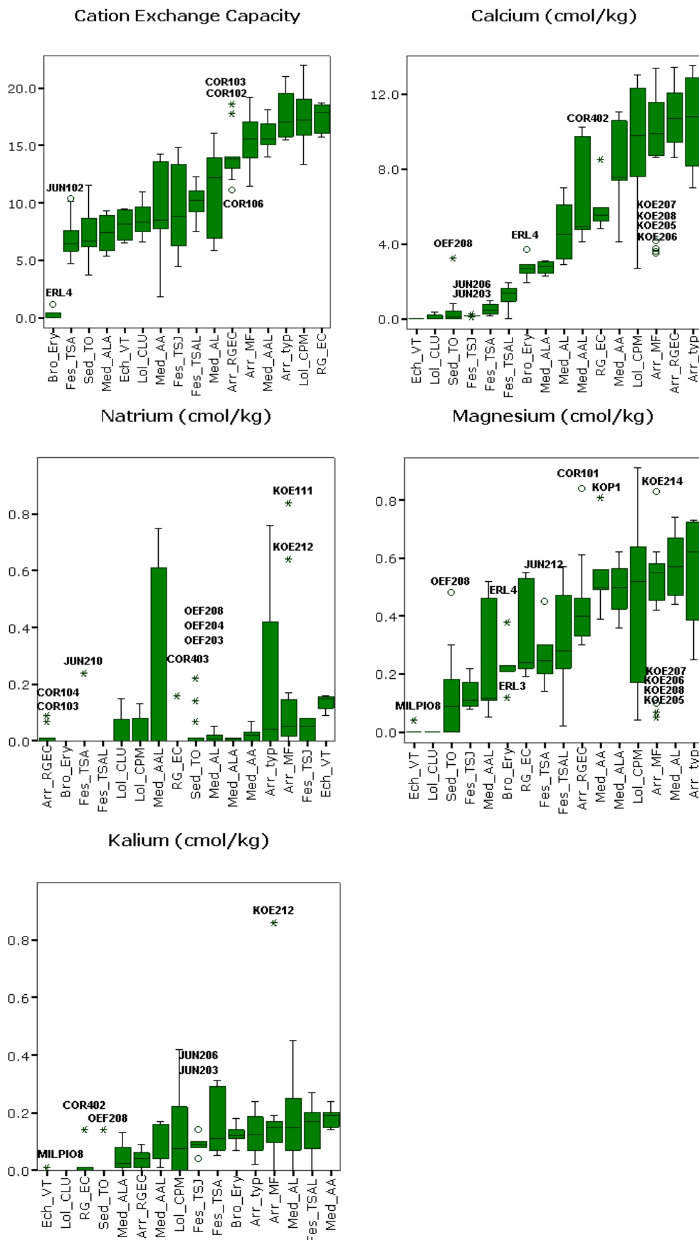
Figuur 2-16 Boxplots met variabelen gerelateerd aan de buffering van de bodem. Kationenomwisselingscapaciteit (C.E.C.), de gemeten basen Calcium (Ca), Magnesium (Mg), Natrium (Na) en Kalium (K). Extreme waarden zijn aangegeven met een asterisk, uitbijters met een cirkel.
