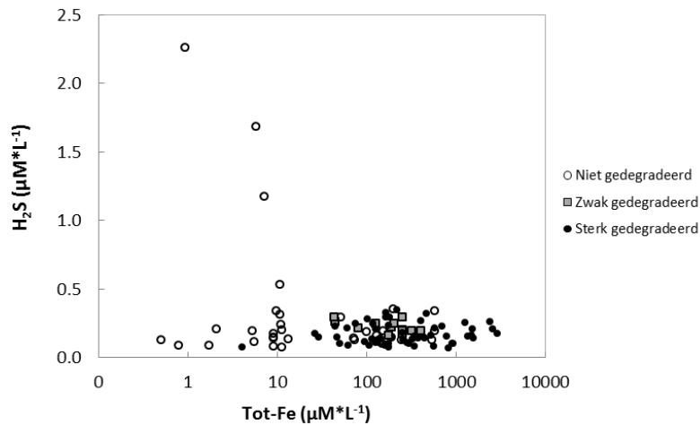
Figuur 32: Sulfideconcentraties uitgezet tegen totaal ijzergehaltes in het porievocht (alle bemonsteringsdieptes).
