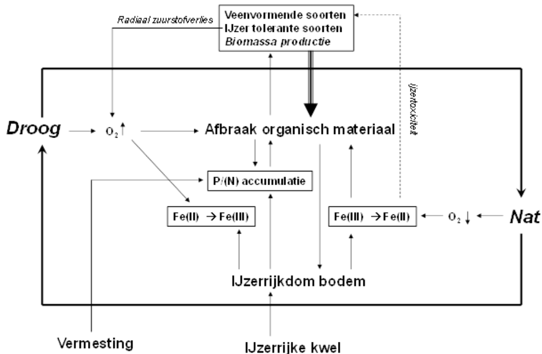
Figuur 5: De invloed van ijzer op de afbraak van veen en accumulatie van N en P.
