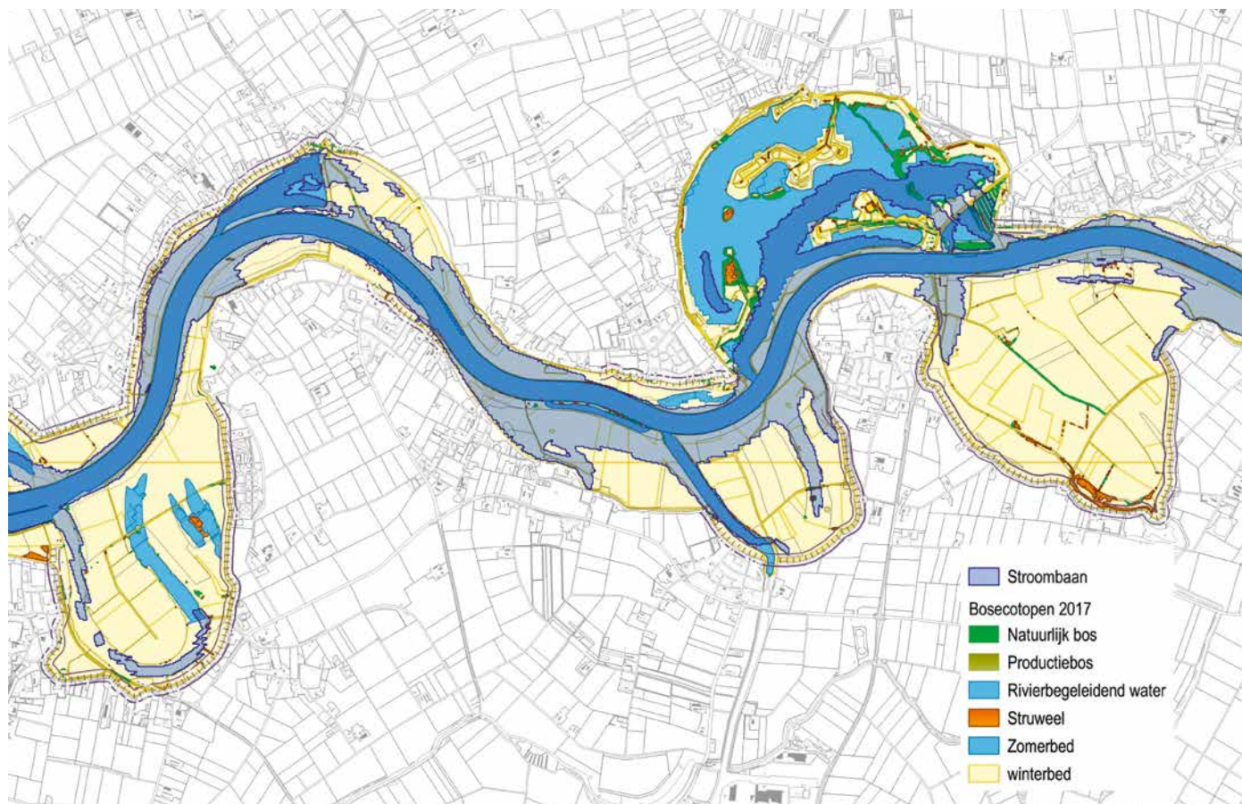
Figuur 14 Delen van de Bedijkte Maas tussen Grave en Lith kennen een smalle stroombaan (definitie project Stroomlijn) dicht op de rivier (blauw) en relatief veel stroomluwe delen in de uiterwaard (geel), waar bos relatief weinig effect heeft op hoogwaterstanden.
