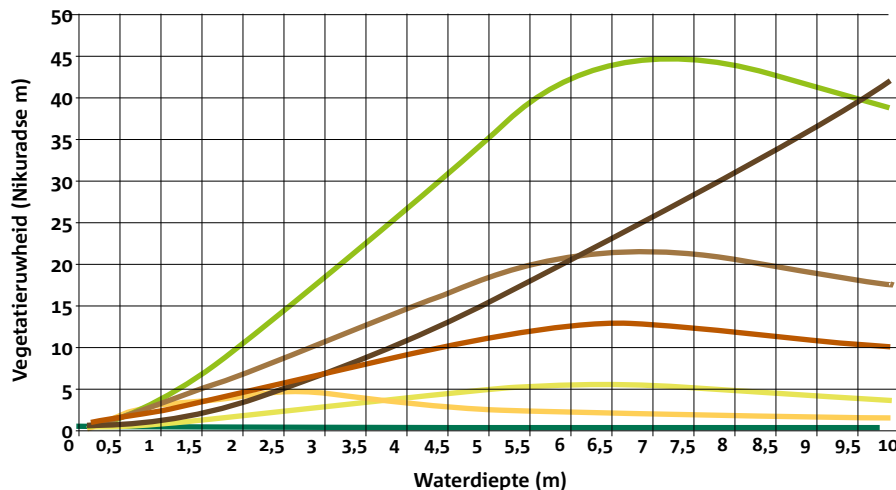
Figuur 13 Hydraulische ruwheid van de verschillende vegetatieklassen uit de vegetatielegger van Rijkswaterstaat.
