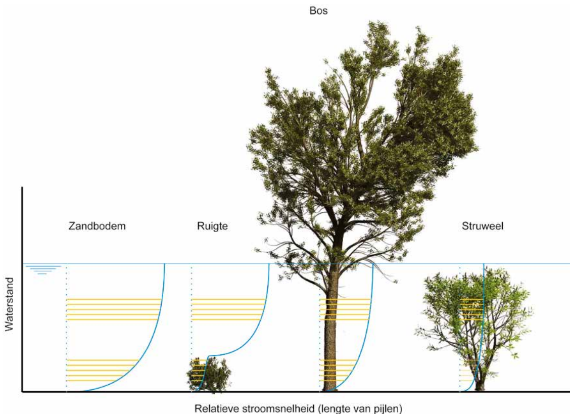
Figuur 10 Schematische weergave van de relatieve stro- mingsweerstand van verschillende vormen ruwe vegetatie (uit Peters e.a., 2006).
