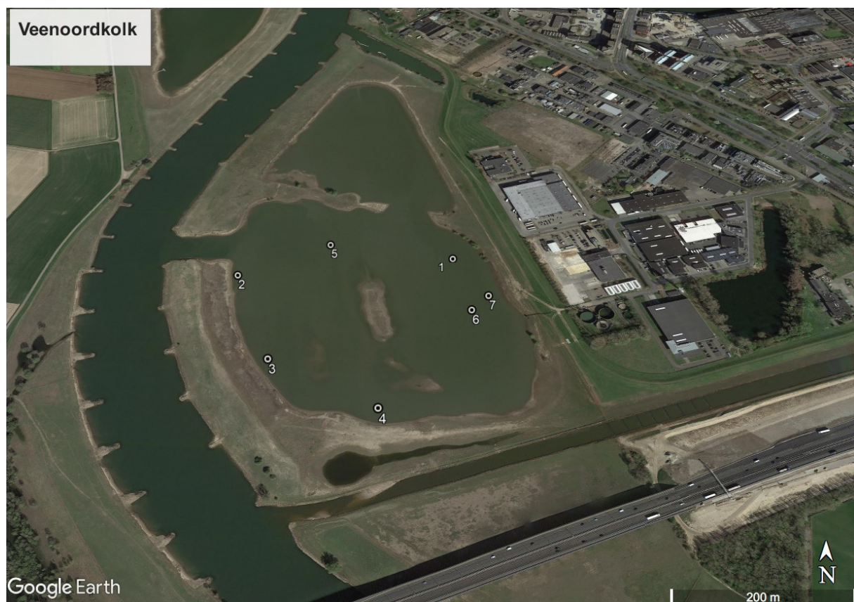
Figuur 49. Overzicht van monster locaties voor bodem- en waterbemonstering.
