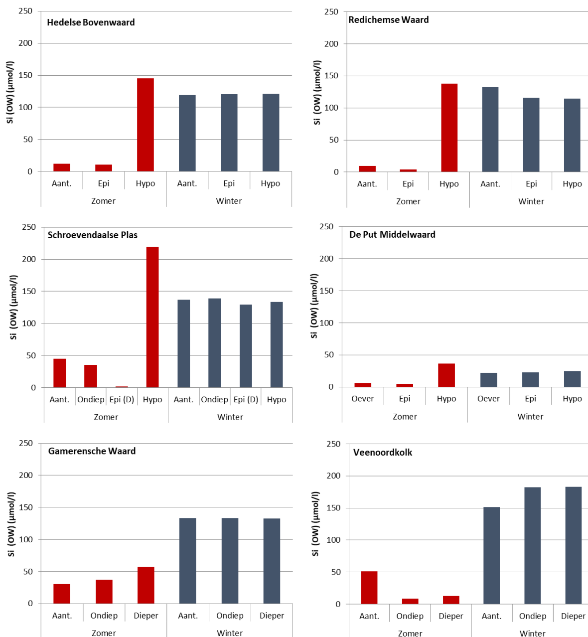
Figuur 86. Siliciumconcentraties ( \mu\text{mol/l} ) in de zomer en winter in het oppervlaktewater van de verschillende plassen.
