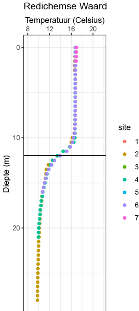
Figuur 62. Temperatuurprofielen van het water op de monsterlocaties.
