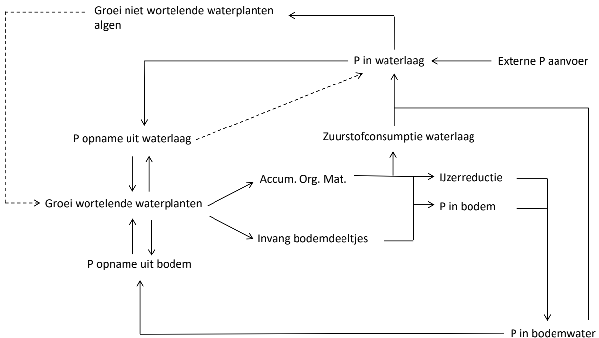
Figuur 5. Schematische weergave van de fosfaatkringloop in een watersysteem.
