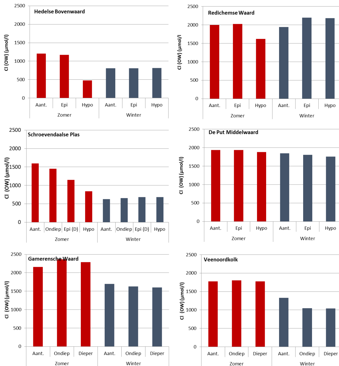
Figuur 85. Chlorideconcentraties ( \mu\text{mol/l} ) in de zomer en winter in het oppervlaktewater van de verschillende plassen.
