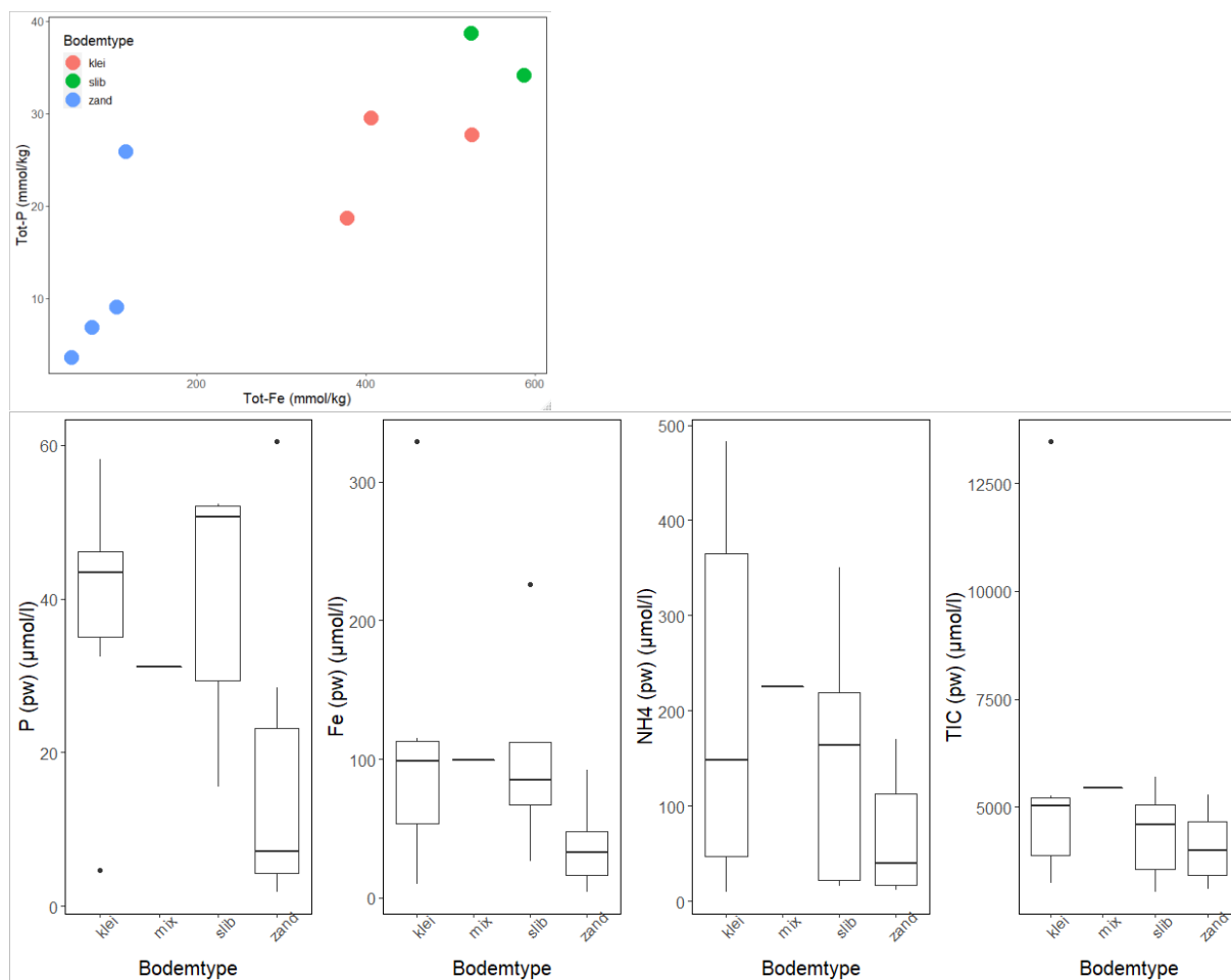
Figuur 57. Boven: Relatie tussen totaal-fosfor en totaal-ijzer (mmol/kg drooggewicht) (zomerwaarden). Onder: Concentratie ( \mu\text{mol/l} ) van fosfor, ijzer, ammonium en anorganisch koolstof in het poriewater (zomer- en winterwaarden) in de verschillende typen bodems.
