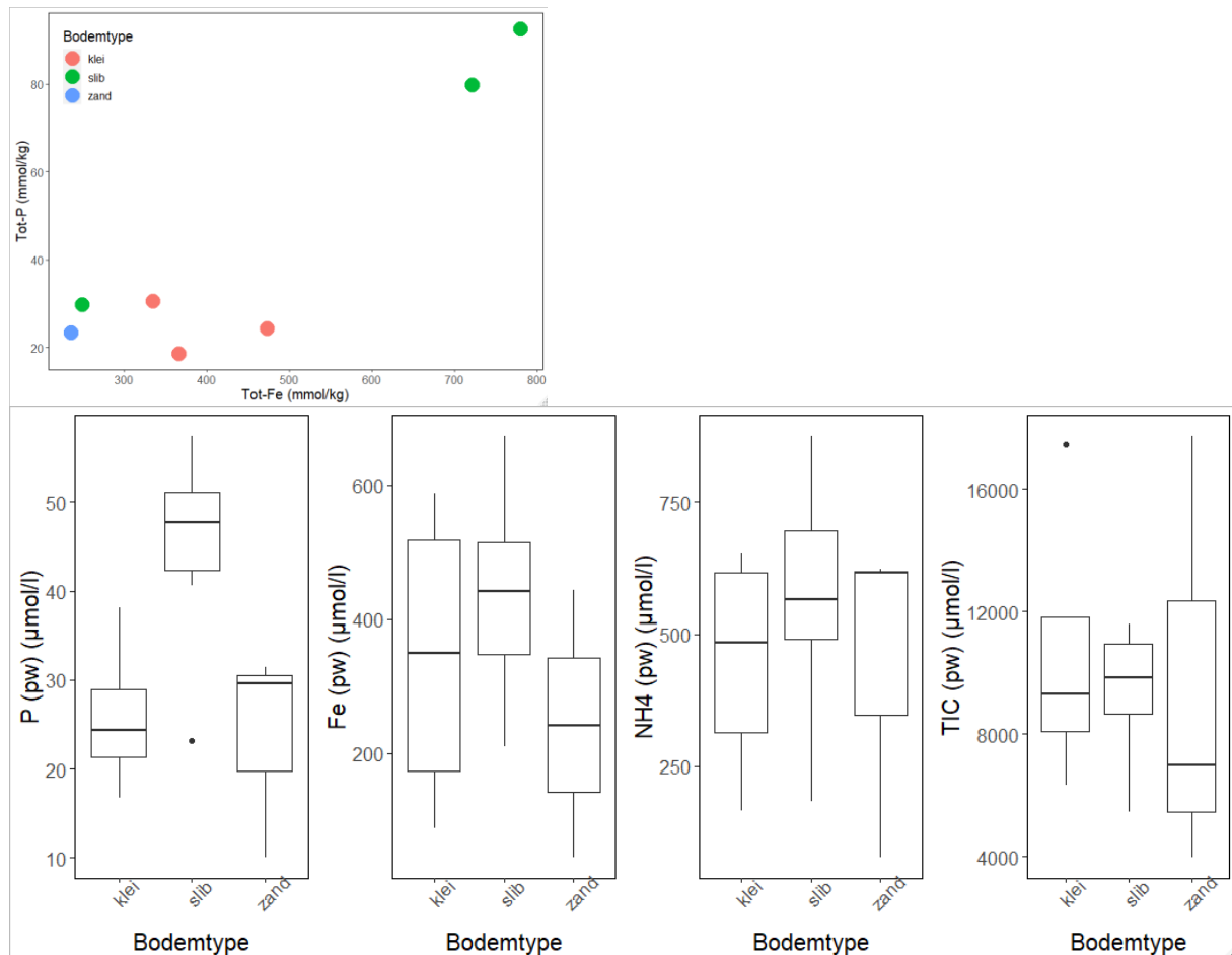
Figuur 75. Boven: Relatie tussen totaal-fosfor en totaal-ijzer (mmol/kg drooggewicht) (zomerwaarden). Onder: Concentratie (μmol/l) van fosfor, ijzer, ammonium en anorganisch koolstof in het poriewater (zomer- en winterwaarden) in de verschillende typen bodems.
