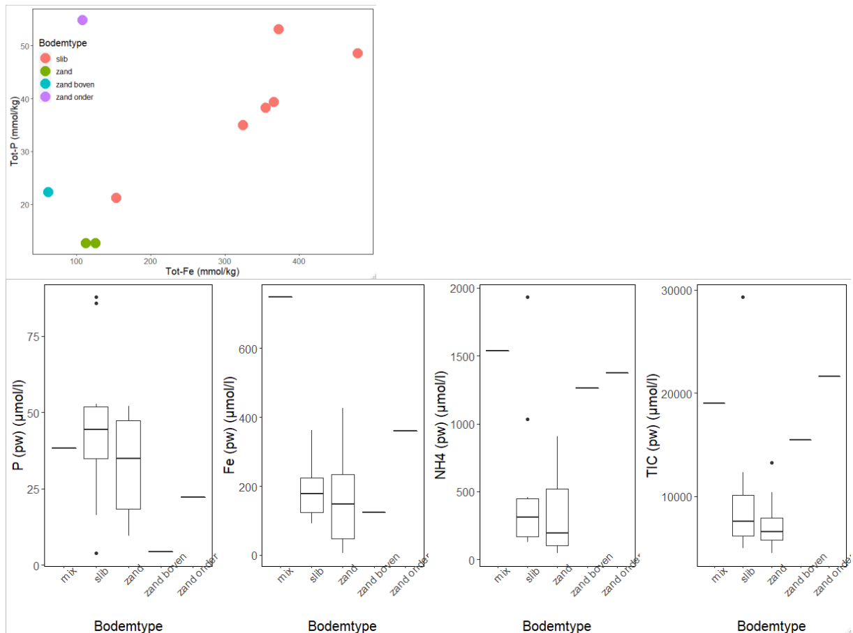
Figuur 51. Boven: Relatie tussen totaal-fosfor en totaal-ijzer (mmol/kg drooggewicht) (zomerwaarden). Onder: Concentratie (μmol/l) van fosfor, ijzer, ammonium en anorganisch koolstof in het poriewater (zomer- en winterwaarden) in de verschillende typen bodems.
