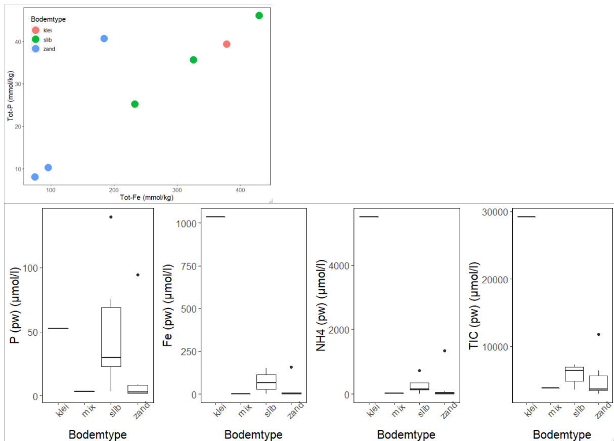
Figuur 69. Boven: Relatie tussen totaal-fosfor en totaal-ijzer (mmol/kg drooggewicht) (zomerwaarden). Onder: Concentratie (μmol/l) van fosfor, ijzer, ammonium en anorganisch koolstof in het poriewater (zomer- en winterwaarden) in de verschillende typen bodems.
