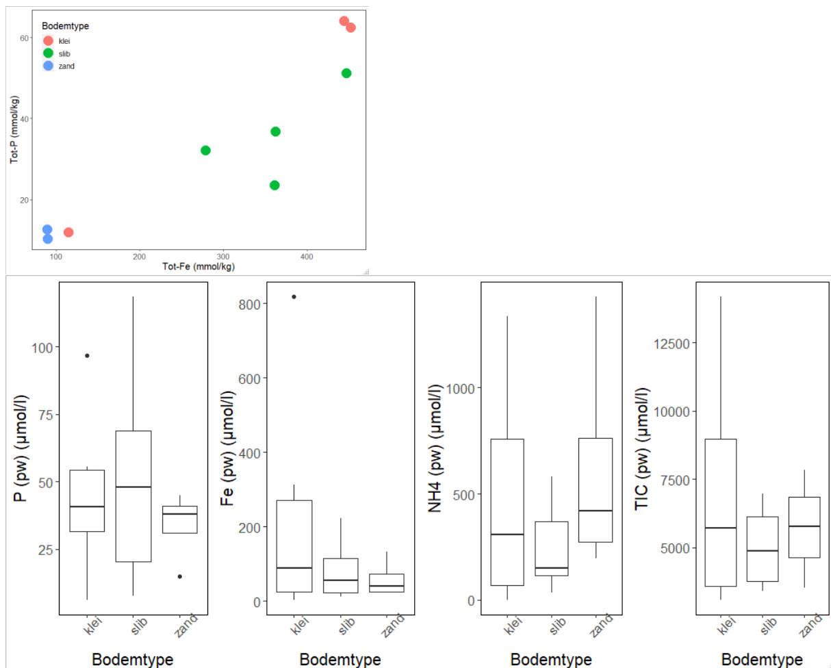
Figuur 63. Boven: Relatie tussen totaal-fosfor en totaal-ijzer (mmol/kg drooggewicht) (zomerwaarden). Onder: Concentratie (μmol/l) van fosfor, ijzer, ammonium en anorganisch koolstof in het poriewater (zomer- en winterwaarden) in de verschillende typen bodems.
