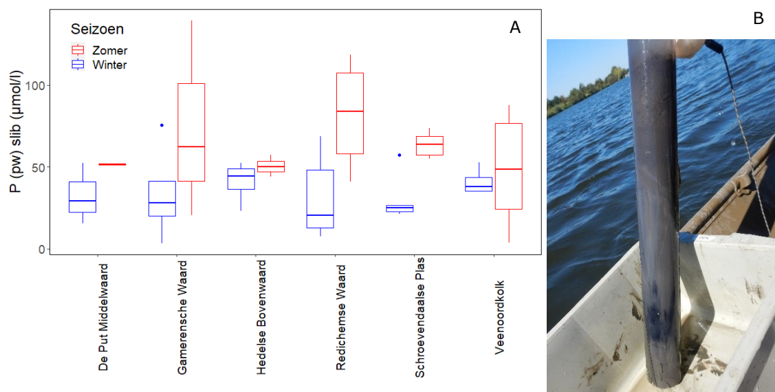
Figuur 27. A: Fosforconcentratie in het poriewater van de slibbodem (μmol/l) van de plassen (in winter en zomer). B: bodemprofiel (Schroeveendaalse plas) met slib in het bovenste deel van de kolom.
