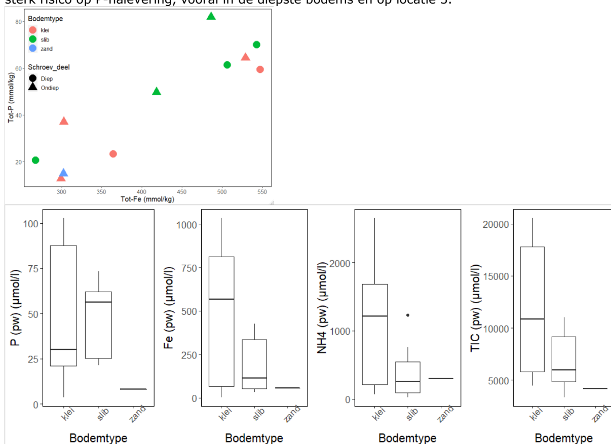
Figuur 81. Boven: Relatie tussen totaal-fosfor en totaal-ijzer (mmol/kg drooggewicht) (zomerwaarden). Onder: Concentratie (µmol/l) van fosfor, ijzer, ammonium en anorganisch koolstof in het poriewater (zomer- en winterwaarden) in de verschillende typen bodems.
