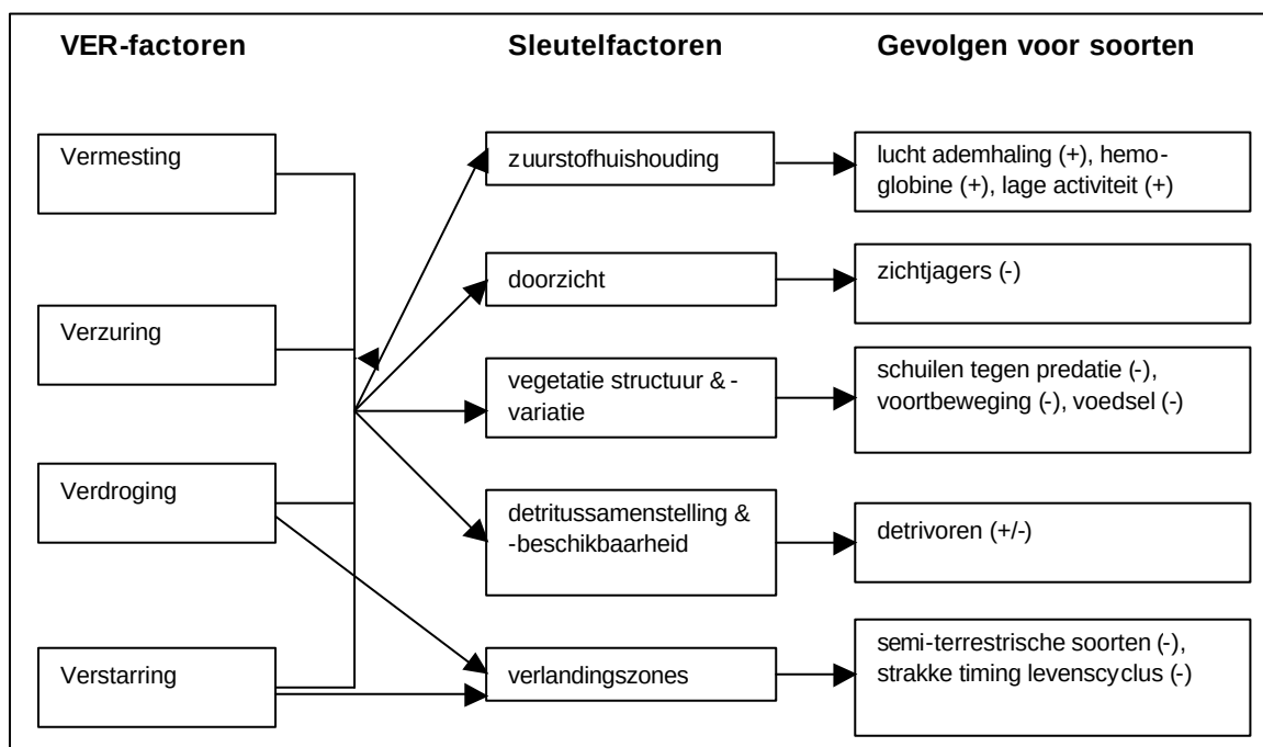
Figuur 10.2 Overzicht van de effecten van aantastingen (VER-factoren) op belangrijke sleutelfactoren (afname of verandering) en bijbehorende veronderstelde gevolgen voor de macrofauna.
