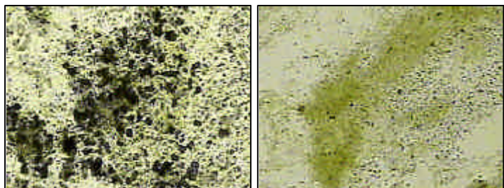
Figuur 9.5 (a) Faeces (l) en Pseudo-faeces (r) A. anatina .
