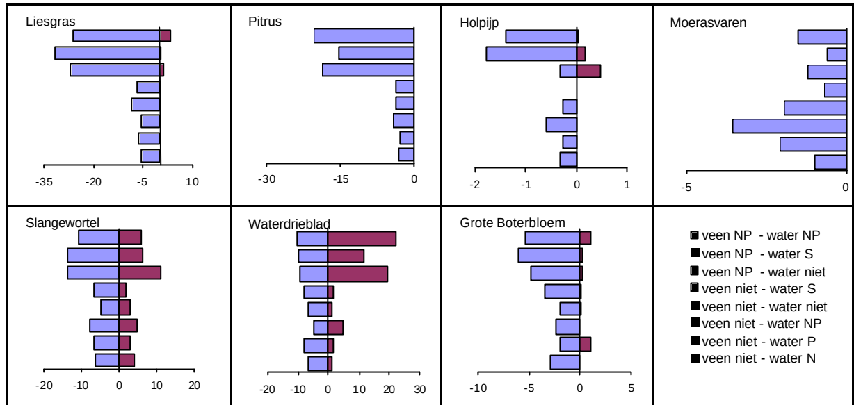
Figuur 4.46 Mate van bedekking van de oever (links) en het water (rechts) door verschillende oeversoorten bij de verschillende bemestingsbehandelingen.
