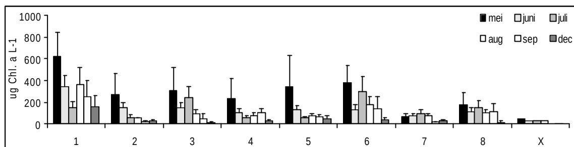
Figuur 4.48 Gemiddelde Chl. a som van alle algen groepen in de 8 behandelingen van het mesocosm experiment in 2005 2 .
