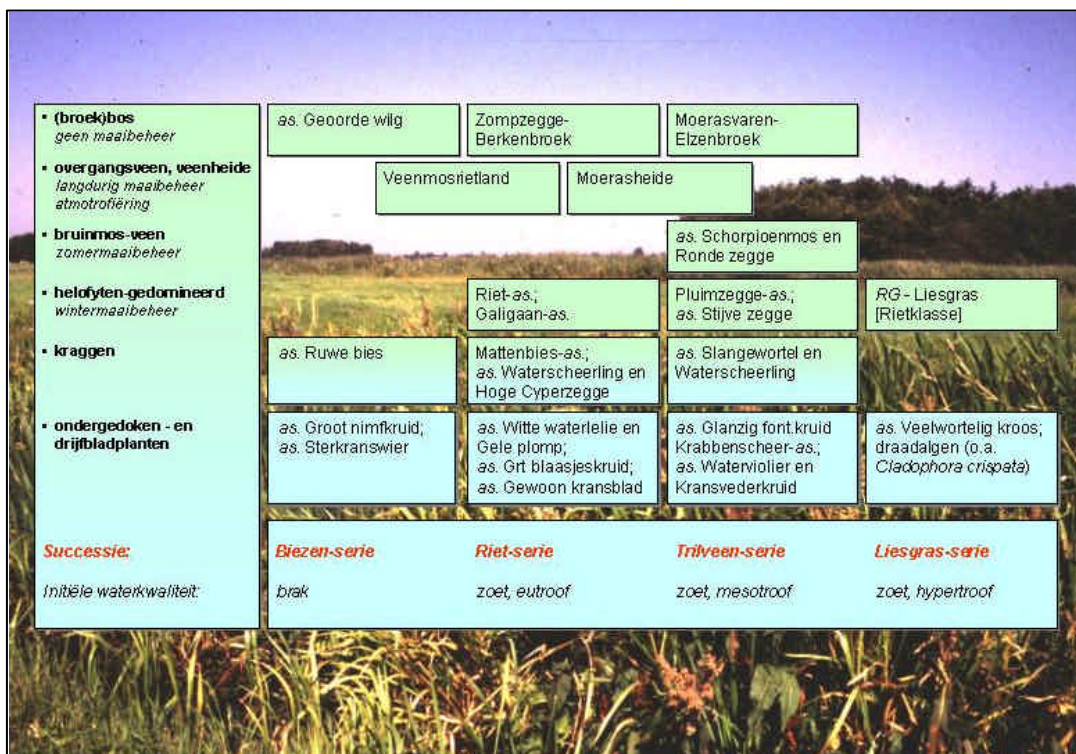
Figuur 2.2 Schema met vegetatiesuccessie-reeksen in laagveenwateren, bij verschillende uitgangssituaties (onderaan weergegeven) en beheerstypen (links weergegeven). Uit: Verhoeven & Bobbink (2001).
