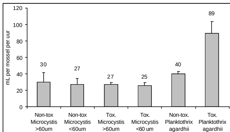
Figuur 9.2 Graas per Dreissena mossel per uur op cyanobacteriën met verschillende vorm en grootte; niet toxische Microcystis (V131) en toxische Microcystis (V40) <60 \mu m en > 60 \mu m, niet toxische P.agardhii (Cya 116) met een gemiddelde lengte van 187mm en toxische P.agardhii (Cya 126) met gemiddelde lengte van 1166mm. (Dionisio Pires et al., 2005).
