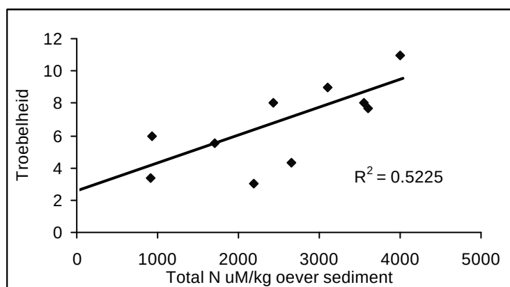
Figuur 4.22 correlatie tussen troebelheid van het petgat water en totale stikstof concentratie per kilo droge stof van de veen oever.
