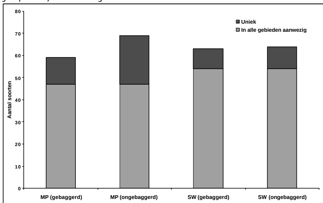
Figuur 10.11 Aantal soorten in de gebaggerde en ongebaggerde delen van de onderzoeksgebieden (voor- en najaar).
