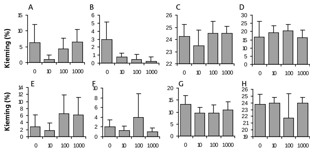
Figuur 8.12 A-H: Kiemingspercentages van verschillende laagveen soorten na 3 weken durende behandeling met 0, 10, 100 of 1000 µM sulfide. A: Watertorkruid ( Oenanthe aquatica ) B: Riet ( Phragmites australis ) C: Moeraszuring ( Rumex palustris ) D: Grote Lisdodde ( Typha latifolia ) E: Hoge cyperzegge ( Carex pseudocyperus ) F: Galigaan ( Cladium mariscus ) G: Gele lis ( Iris pseudacorus ) H: Grote kattenstaart ( Lythrum salicaria ).
