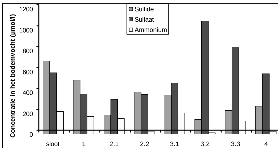
Figuur 5.14 Concentraties sulfide, sulfaat en ammonium in het bodemvocht in een isolatie gradiënt van petgaten in het Ilperveld.
