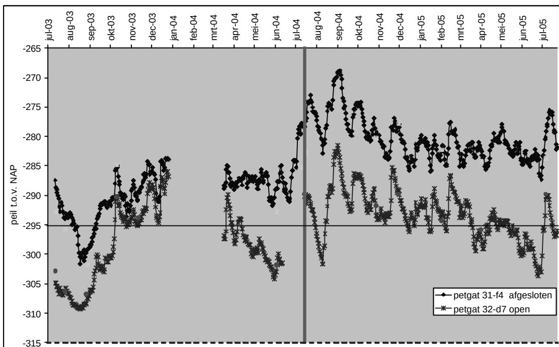
Figuur 5.5b Waterpeil in de nieuwe, noordelijk gelegen petgaten in Westbroek. De horizontale lijnen geven de hoogte van de afvoerbuizen aan (donker = 31-f4, onderbroken = 32-d7). De verticale dubbele lijn geeft aan wanneer petgat 31-f4 is afgesloten. Losse stippen zijn handmetingen.
