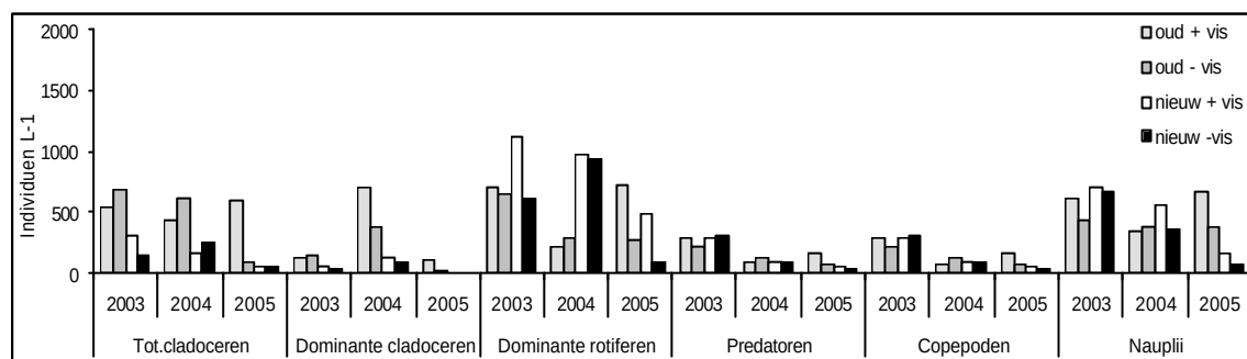
Figuur 4.32 Belangrijkste zoöplankton groepen in De Deelen (2003-2006).
