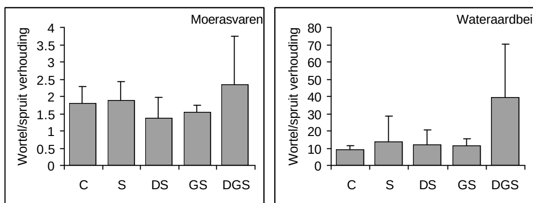
Figuur 8.8 Verschillen in wortel/spruit verhouding van moerasvaren en wataardbei voor de verschillende behandelingen.
