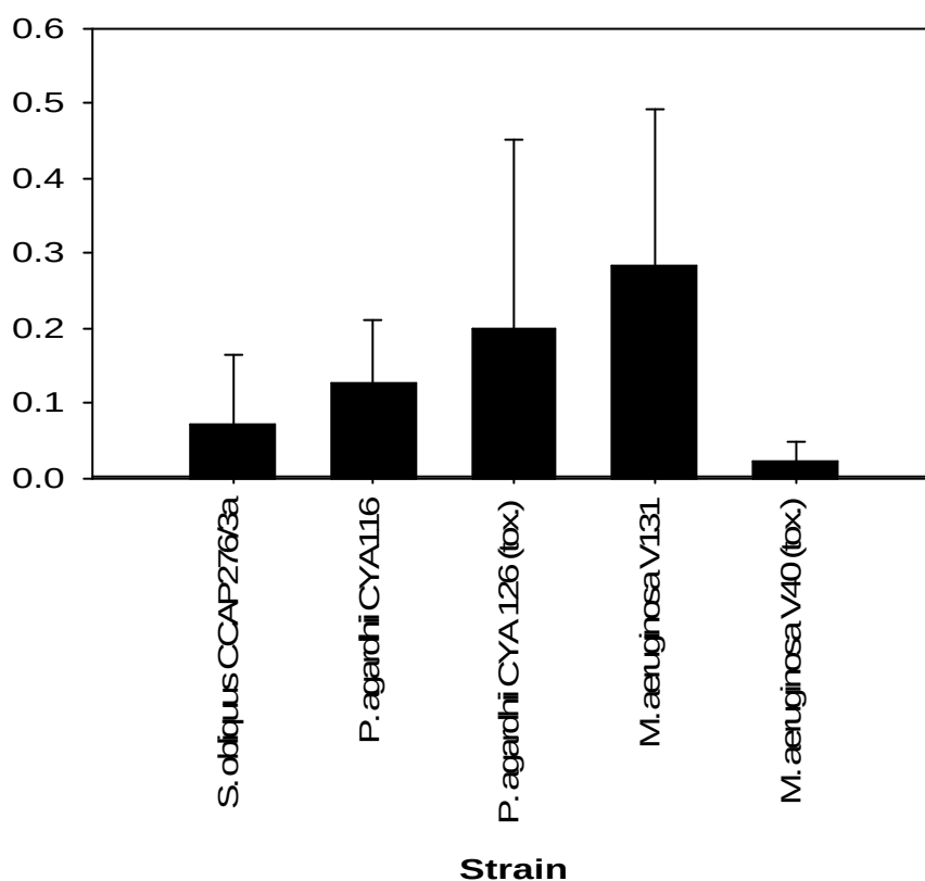
Figuur 9.11 Pseudo-faeces productie als fractie berekend van het totale volume dat schoongezeefd is van algen (CR).
