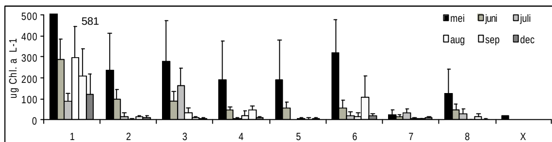
Figuur 4.49 Gemiddelde groenalgen biomassa in de 8 behandelingen van het mesocosm experiment in 2005 1 .
