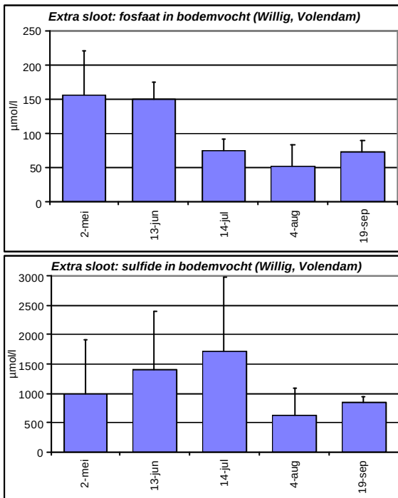
Figuur 5.17 Fosfaat- en sulfideconcentraties in een boerensloot in Volendam in de zomer van 2003. De sloot viel vanaf eind juni vrijwel droog.
