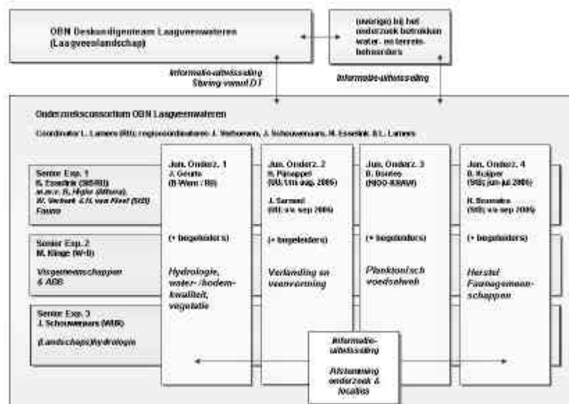
Figuur 2.7 Organisatieschema voor het onderzoek ten behoeve van OBN-Laagveenwateren; laatste jaar van fase 1
