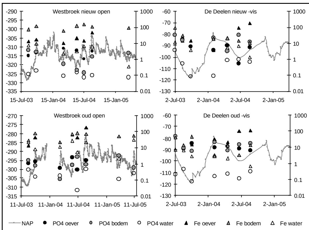
Figuur 5.10 Peilverloop (linkeras, cm NAP) en fluctuaties in concentraties (rechteras, \mu\text{M} ) fosfaat (cirkels) en ijzer (driehoekjes) in oevervocht, waterbodenvocht en oppervlaktewater in petgaten in Westbroek en De Deelen.
