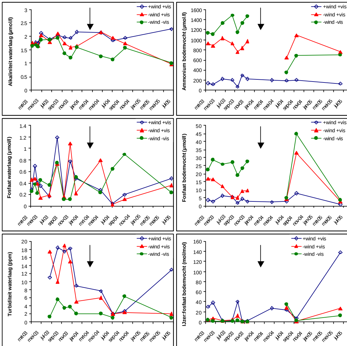
Figuur 6.9 Ontwikkeling van de watersamenstelling (links) en de bodemvochtsamenstelling (rechts) in de petgaten in Terra Nova, na afwisseling in de winter van 2002/2003. De pijl geeft aan wanneer ook het petgat +wind +vis afgevisst werd, in de winter van 2003/2004.
