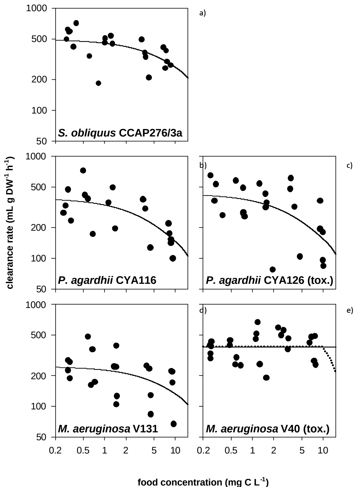
Figuur 9.8 De CR (Clearance Rate); dit is de snelheid waarmee A. anatina het medium ontdoet van de algen (weergegeven in ml per gram drooggewicht per uur). Deze waarden zijn nog niet gecorrigeerd voor evt. uitgescheiden pseudo-faeces (nog niet verteerde algen). Voor meer kenmerken en uitleg over de gebruikte algen zie Bijlage 17.
