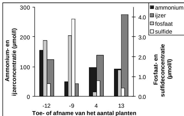
Figuur 7.7 Vergelijking tussen de toe- of afname van het aantal Krabbenscheerplanten in de vier Wapserveense petgaten en de ammonium-, ijzer-, fosfaat- en sulfideconcentraties in het onderwaterbodenvocht.
