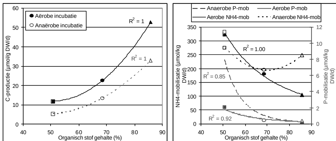
Figuur 7.14 Een vergelijking tussen Nederlandse waterbodems (■; n=30 ), Ierse waterbodems (□; n=12 ) en Ierse kraggebodems (△; n=42 ). Links de relatie tussen organisch stofgehalte en decompositiesnelheid. Rechts de relatie tussen organisch stofgehalte en mineralisatiesnelheid.
