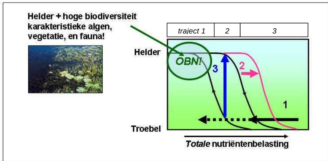
Figuur 11.2 Alternatieve toestanden (helder met onderwaterplanten, versus troebel of met kroosdek/flab) in laagveenwateren afhankelijk van de nutriëntenbelasting (met name P), hysteresis-effect, en de ligging van het uiteindelijke OBN-doel, een hoge biodiversiteit. Echter, alle aangegeven maatregelen, in alle drie de trajecten, kunnen in principe binnen het kader van OBN gebruikt worden, ook bij minder ambitieuze doelen. Maatregelen in plassen zullen bovendien doorwerken in de 'haarvaten' (sloten, petgaten) van het systeem, die vrijwel altijd hogere herstelkansen hebben. Mogelijke maatregelen: 1. brongerichte maatregelen: zowel externe als interne bronnen; 2. maatregelen die de kritische belasting verhogen; 3. maatregelen voor omslag door ingreep in trofische interacties (ABB). Naar Klinge, schriftelijke mededeling. Voor overige uitleg, zie tekst.
