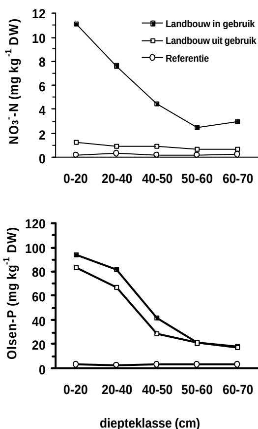
Figuur 11.11 Waarden voor geëxtraheerd nitraat en fosfor in diepteprofielen van landbouwgrond, voormalige landbouwgrond (natuurontwikkeling) en een natuurlijke referentiebodem in een schraalland.
