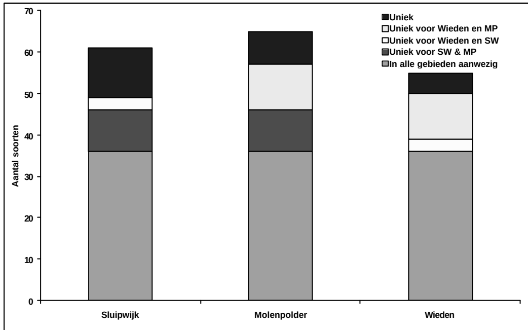
Figuur 10.10 Aantal soorten in de verschillende gebieden (najaar). Er is onderscheid gemaakt tussen unieke en niet unieke soorten voor een gebied. Tevens is een onderverdeling gemaakt waarbij soorten in twee van de drie gebieden voorkomen.
