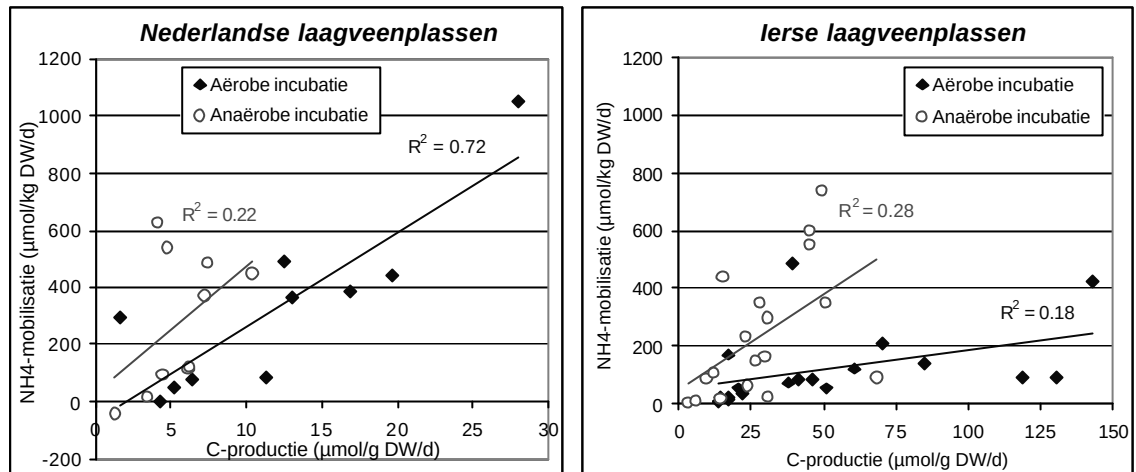
Figuur 7.13 Correlatie tussen ammoniummobilisatie en C-productie (decompositie) tijdens aërobe en anaërobe incubatie van Nederlandse en Ierse laagveenbodems ( n=3 ).
