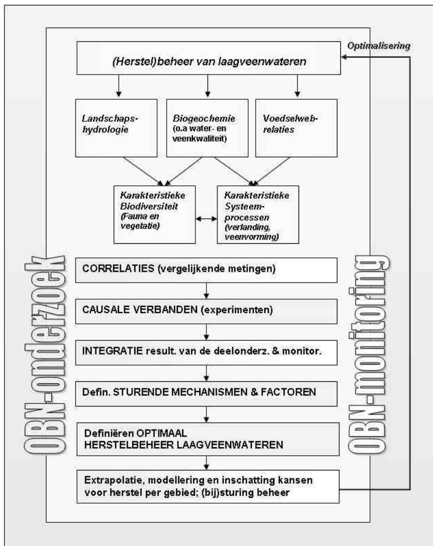
Figuur 2.6 Schematische onderzoeksopzet OBN-Laagveenwateren
