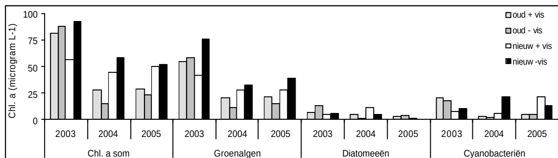
Figuur 6.19 Gemiddelde Chl. a concentraties van de groepen algen in De Deelen in 2003, 2004 en 2005.
