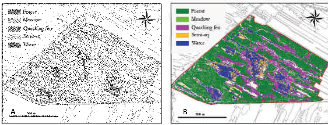
Figuur 8.13 Resultaten van de classificatie van luchtfoto's van het Hol van 2000 (A) en 2003 (B).
