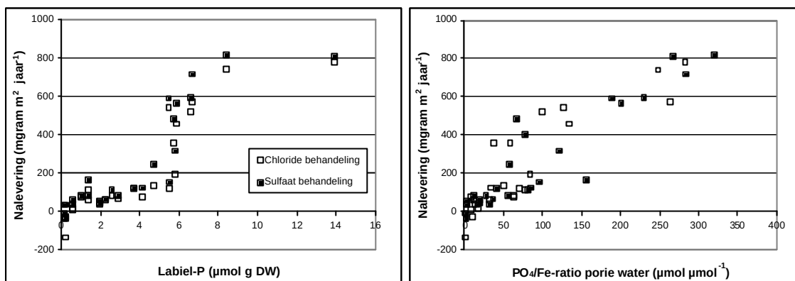
Figuur 4.16 Relaties tussen de nalevering, de Labeil-P fractie van het sediment en de PO 4 /Fe ratio van het bodemvocht na toediening van chloride (4 mM) of sulfaat (2 mM) in het bovenstaande water.
