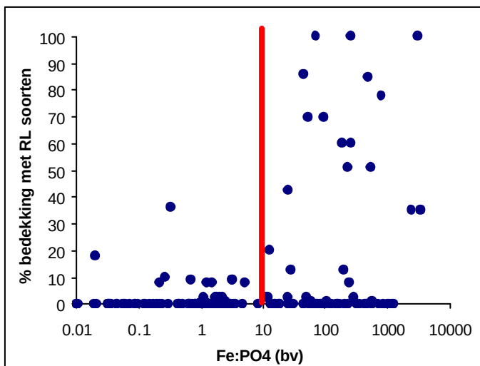
Figuur 4.11 Relatie tussen de ijzer:fosfaat ratio in het onderwaterbodenvocht en de bedekking van de waterlaag met Rode Lijst-soorten, mesotrafente soorten en eutrafente soorten (indeling gebaseerd op Bloemendaal & Roelofs, 1998; soortenlijst in Bijlage 8).
