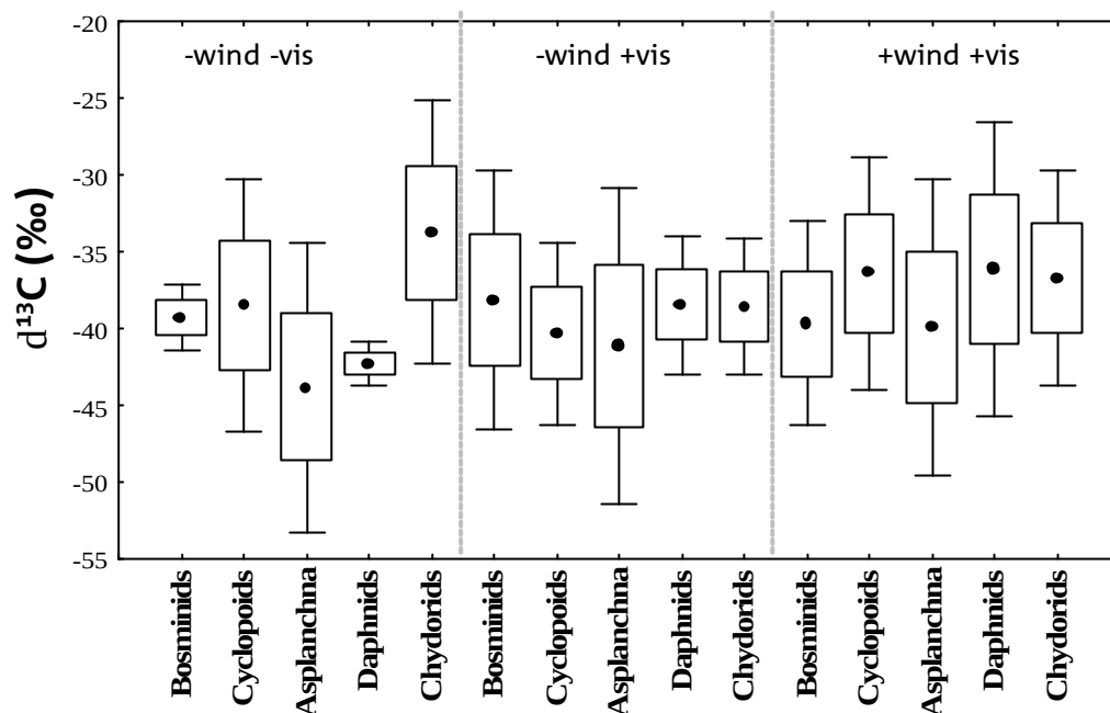
Figuur 6.16 (b) d^{13}C waarden van de belangrijkste zoöplankton groepen in de 3 behandelingen.
