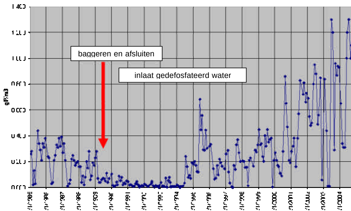
Figuur 11.10 Verloop van de fosfaatconcentratie ( \text{mg PO}_4\text{-P/l} ) in het oppervlaktewater van de Geerplas (Zuid-Holland) na baggeren. Gegevens B.. Michielse, Hoogheemraadschap van Rijnland.
