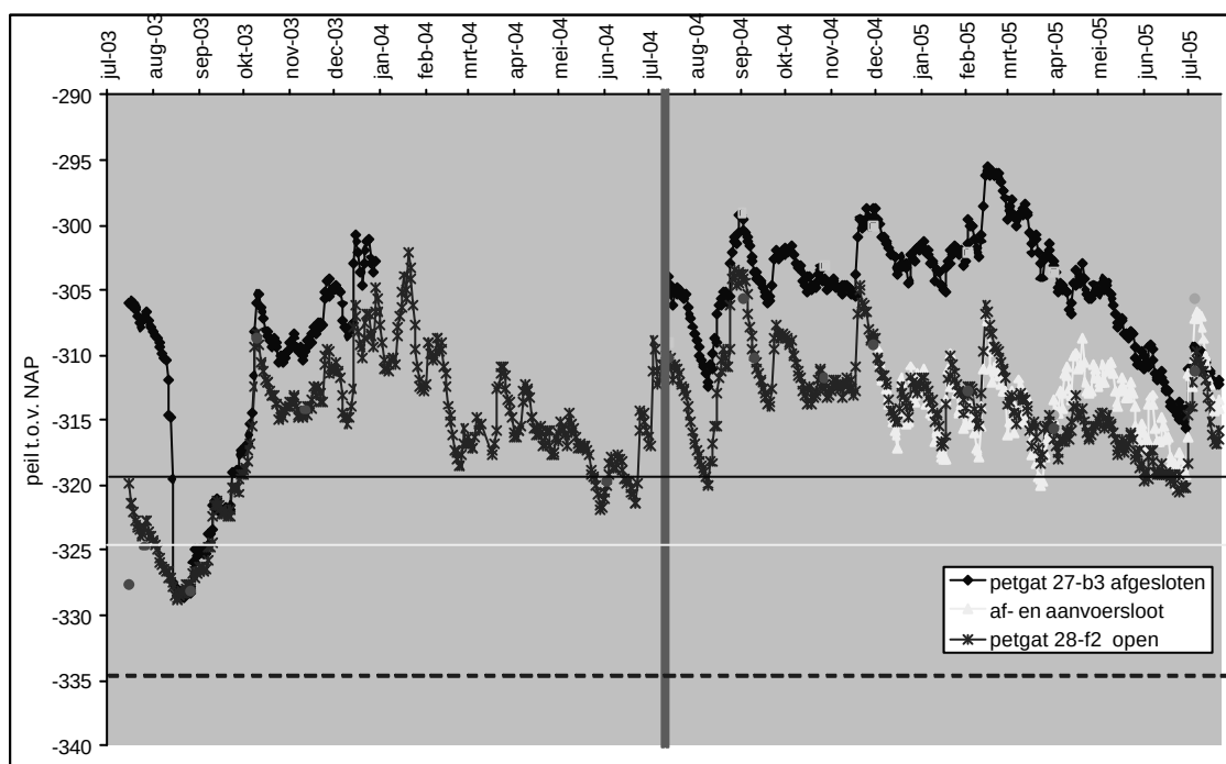
Figuur 5.5a Waterpeil in de oude, zuidelijk gelegen petgaten in Westbroek, en in de sloot waarop beide petgaten normaliter afvoeren. De horizontale lijnen geven de hoogte van de afvoerbuizen aan (donker = 27-b3, onderbroken = 28-f2, licht = sloot t.h.v. 28-f2). De verticale dubbele lijn geeft aan wanneer petgat 27-b3 is afgesloten. Losse stippen zijn handmetingen.
