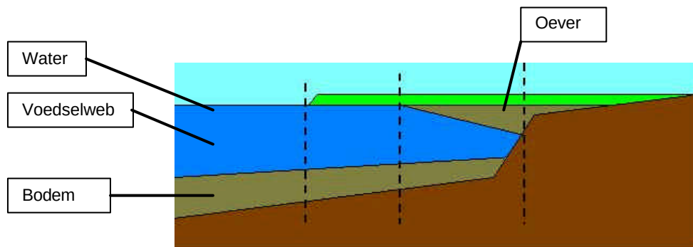
Figuur 4.1 Schematische weergave van een ideale verlanding en de verschillende componenten die bemonsterd zijn door de verschillende junior onderzoekers.
