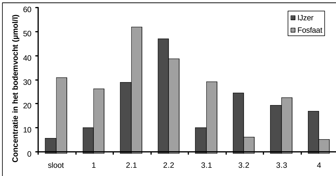
Figuur 5.15 Concentraties ijzer en fosfaat in het bodemvocht in een isolatie gradiënt van petgaten in het Ilperveld.
