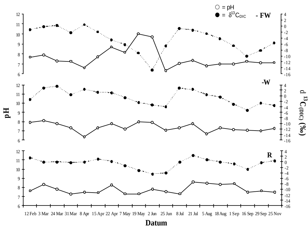
Figuur 6.15 pH en de d^{13}C waarde (= ratio van ^{13}C vs. ^{12}C in vetzuren) van de koolstof bron voor fytoplankton groei. -FW = -wind -vis, -W = -wind +vis, R = +wind +vis. Effecten visbeheer op isotoop waarde van opgelost anorganisch koolstof (DIC), fyto- en zoöplankton
