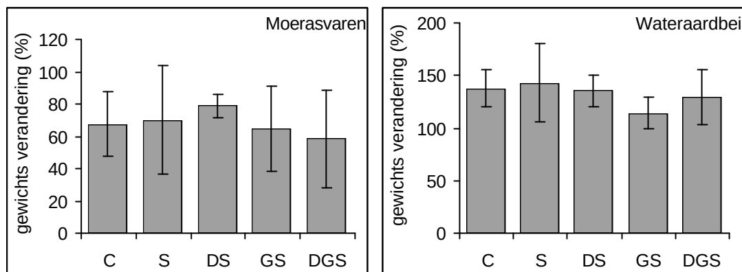
Figuur 8.7 Verandering in drooggewicht van Moerasvaren en Wataardbei voor de verschillende behandelingen. Letters indiceren de verschillende licht behandelingen C: Controle, direct daglicht, S: Enkele laag Schaduwdoek DS: Dubbele laag schaduwdoek, GS: Groene Schadu, één laag filterpapier, DGS: Dubbele laag groen filterpapier (zie ook Tabel 8.2).
