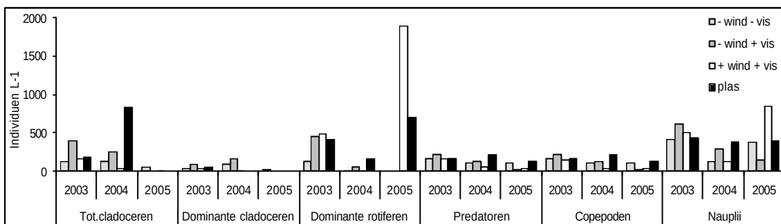
Figuur 4.35 Belangrijkste zoöplankton groepen in Terra Nova (2003-2006).
