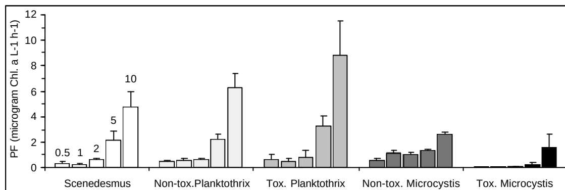
Figuur 9.10 Pseudo-faeces productie door Anodonta anatina (mg Chl. a per liter per uur) na 60 minuten gegraasd te hebben op 5 algen (1 groen alg + 4 blauw algen) in 5 concentraties (0.5-1-2-5 en 10 mg koolstof per liter medium).
