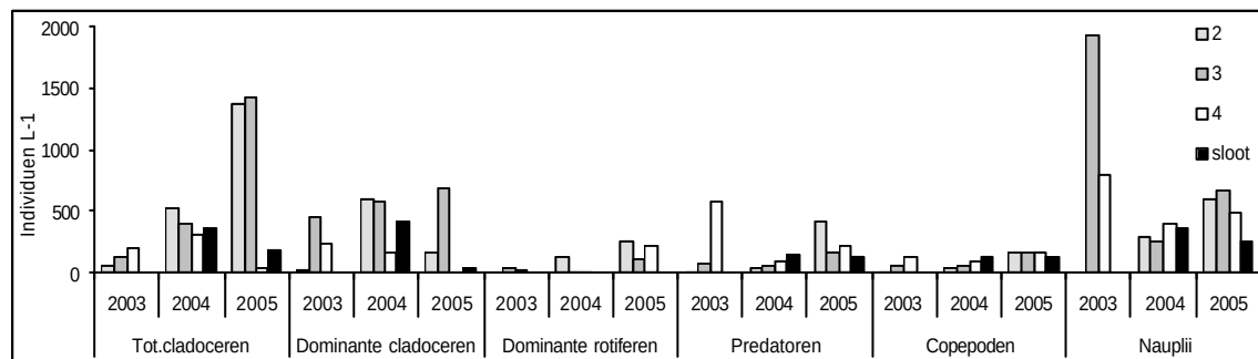
Figuur 4.34 Belangrijkste zoöplankton groepen in IJperveld (2003-2006).
