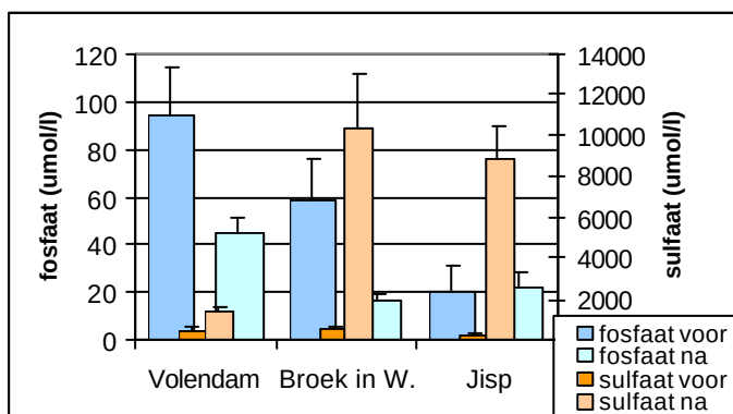
Figuur 5.18 Fosfaat- en sulfaatconcentraties voor en na het verdrogen van de bodems in het laboratorium.
