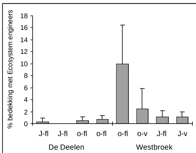
Figuur 5.12: Bedekkingspercentages van kraggenvormende ecosystem engineers in de verschillende petgaten in Westbroek en De Deelen. J: jonge petgaten, o: oude petgaten. Fl: met een fluctuerend peil (geïsoleerd), v: met een vast peil (open).
