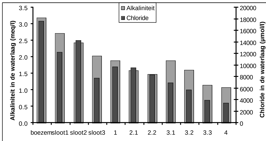
Figuur 5.13 Chlorideconcentratie en alkaliniteit in een isolatie gradiënt van petgaten in het Ilperveld.
