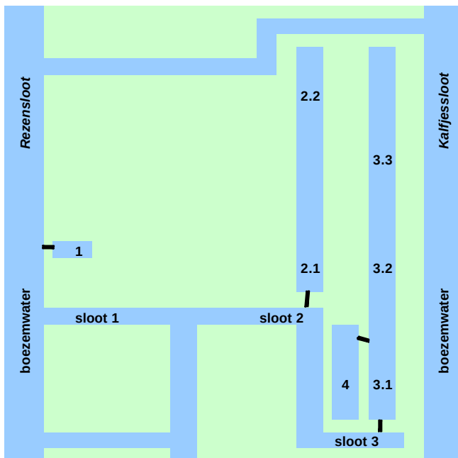
Figuur 5.3 Schematische weergave van de ligging van de onderzochte petgaten in het IJperveld, waarbij een hoger getal een meer geïsoleerde ligging aangeeft.
