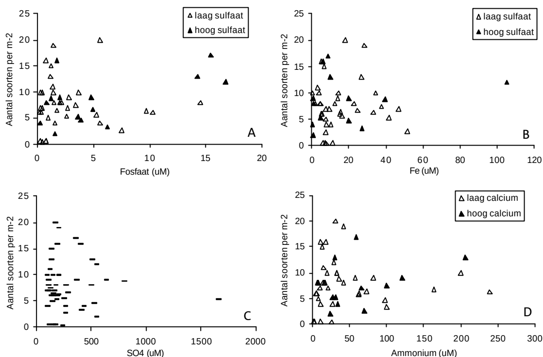
Figuur 4.19 Relatie tussen het aantal soorten per m 2 en fosfaat (A), ijzer (B), sulfaat (C) ammonium (D).
