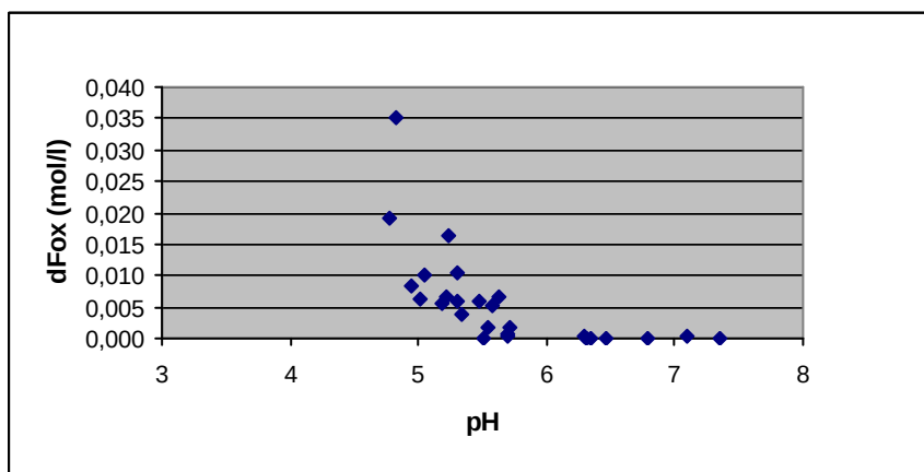
Figuur 15 Verband tussen pH en het verlies aan fosfaatadsorptiecapaciteit door het oplossen van ijzeroxiden bij een daling van de redoxpotential van pe=3 naar pe=-3 (alle standplaatsen m.u.v. Ilperveld).
