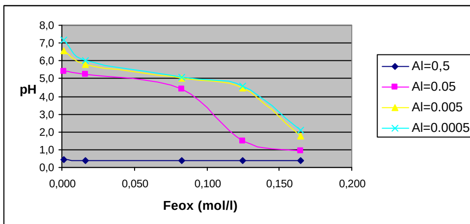
Figuur 6 Invloed van het ijzeroxidegehalte op de pH bij verschillende aluminiumoxidegehalten
