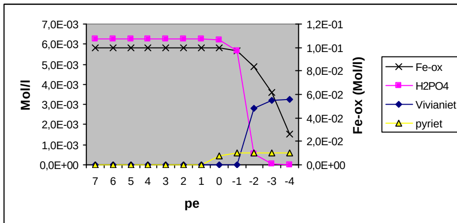
Figuur 13 Het verloop van de fosfaatconcentratie, de vorming van pyriet en vivianiet en het oplossen van ijzeroxide bij daling van de redoxpotential ervan uitgaande dat al het fosfaat in de aërobe fase in opgeloste vorm aanwezig zou zijn (Tr19-Oh).
