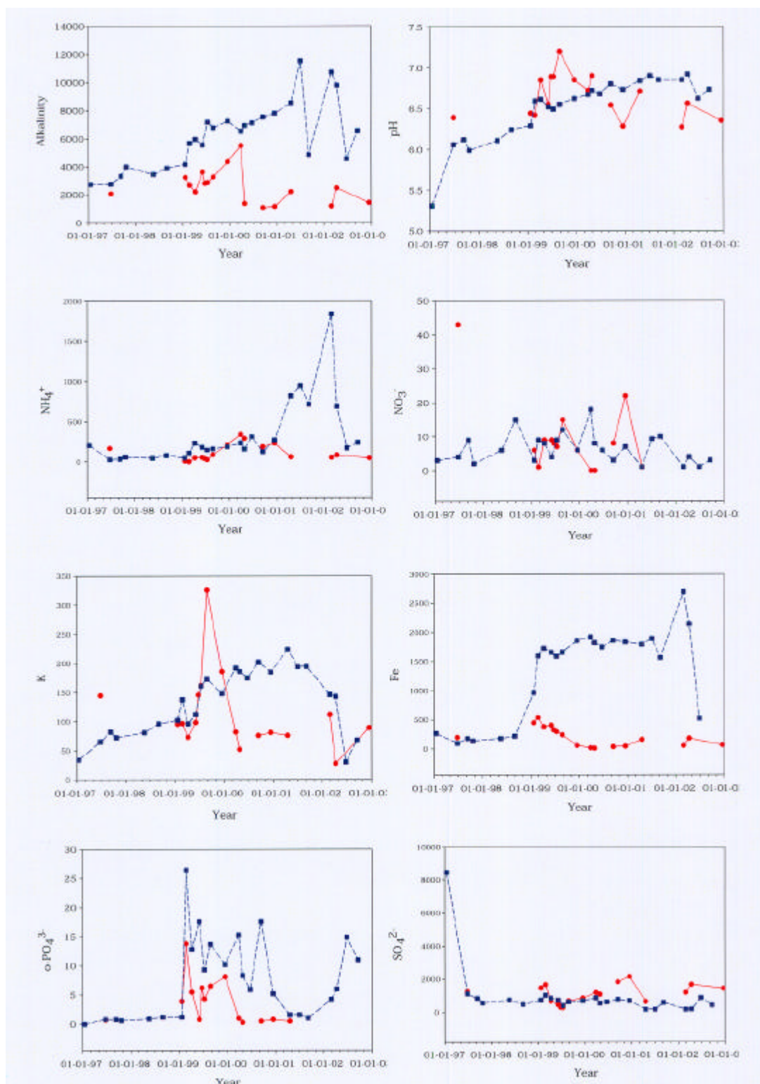
Figuur 3. 16. De concentratie in het oppervlakte water (?) en bodemvocht (l) van plot 21. Alkaliniteit in [ \mu\text{eq.l}^{-1} ] en concentraties in [ \mu\text{M} ]
