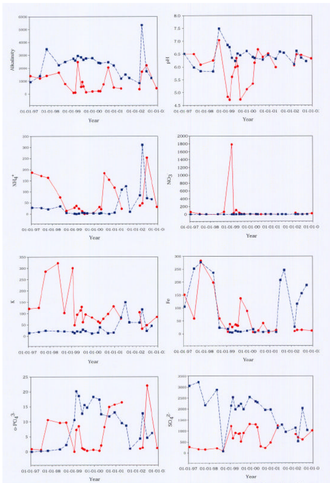
Figuur 3. 20. De concentratie in het oppervlakte water (.) en bodemvocht (.) van plot 61. Alkaliniteit in [ \mu\text{eq. l}^{-1} ] en concentraties in [ \mu\text{M} ]
