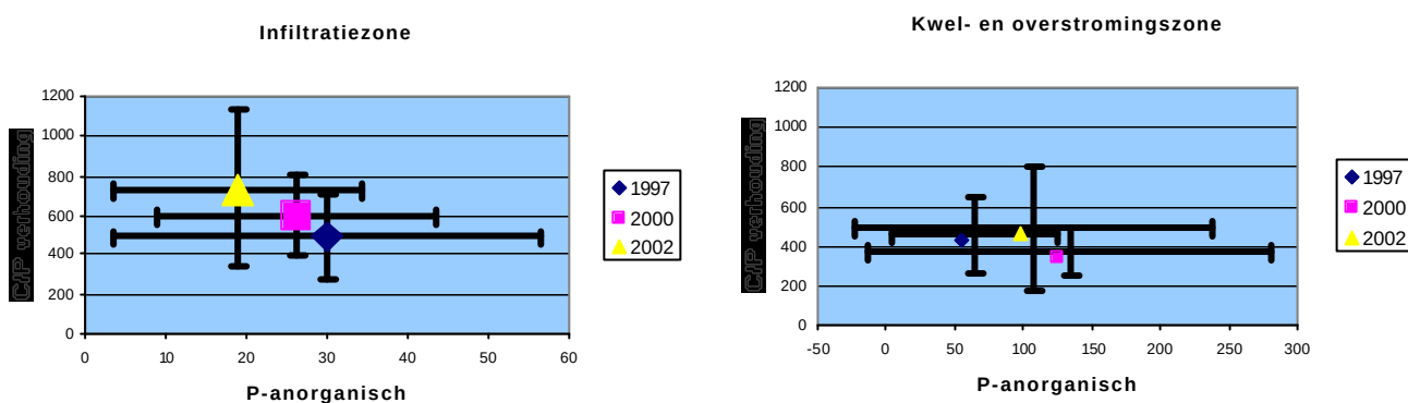
Figuur 4. 4. Gemiddelde waarden en standaardafwijking van de C/P verhouding en het anorganisch fosfaatgehalte in de twee deelgebieden van Koelbroek in 1997, 2000 en 2002.
